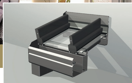
TD BUITENLIGGENDE STATICA
