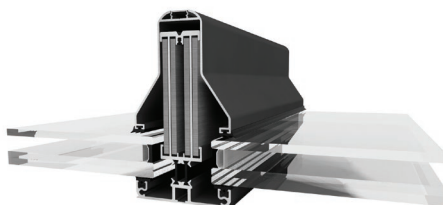
Chevron épine à capot
