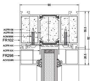
FR90 vaste wand EI60
