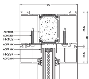
FR90 vaste wand EI30
