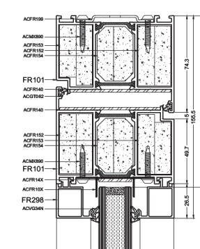
FR90 deur EI60
