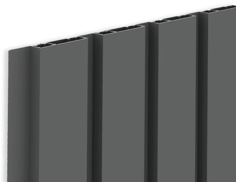
DW240 ist ein vertikales Abschluss-Profil von 80 mm Breite. Damit werden die vertikalen Linien nicht so stark betont. Ideal für größere Flächen.
