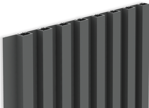
DW230 ist ein flaches vertikales Abschluss-Profil. Profil-Maß: Breite 30 mm, Tiefe 20mm.
