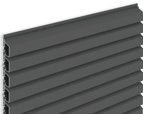
DW233 ist ein horizontales Abschluss-Profil. Die abfallende Spitze stellt sicher, dass sich kein Wasser auf den Profilen ansammelt.
