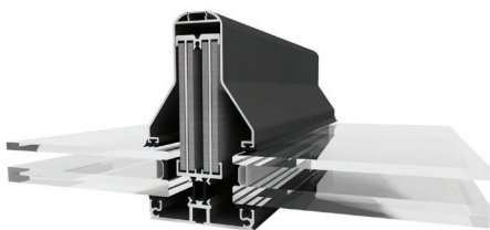
Buitenliggende statica met afdekkap
